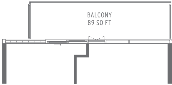
UNIT 601
