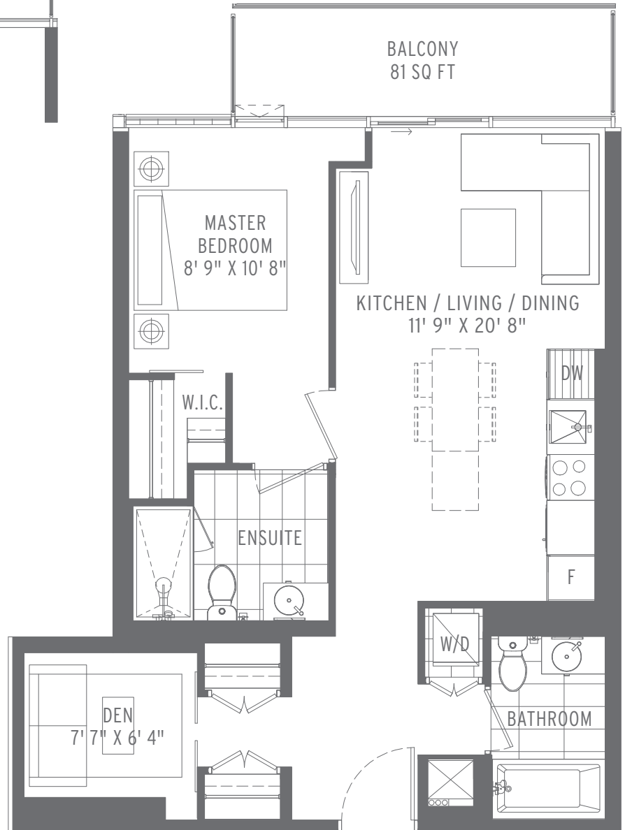
UNITS 701, 801, 901, 1001 & 1101
